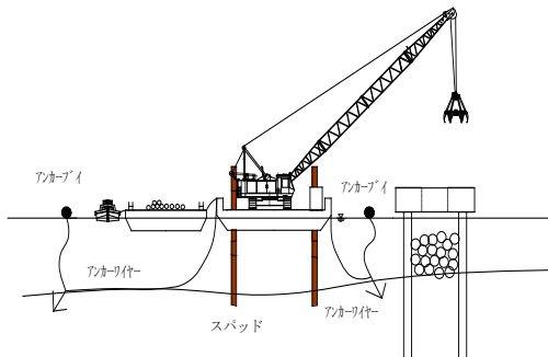
詰石投入
