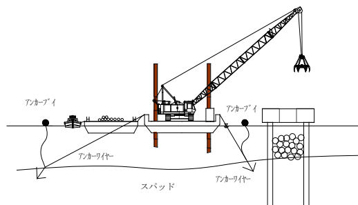
台船移動時
