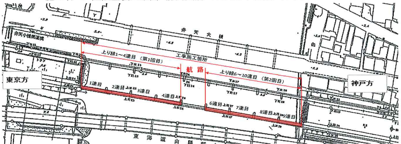
足場概略図
