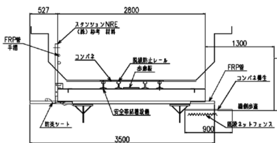
足場断面図
