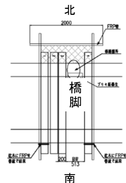
足場平面図
