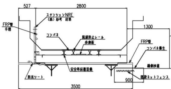
足場断面図
