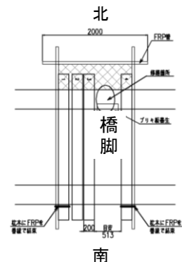
足場平面図
