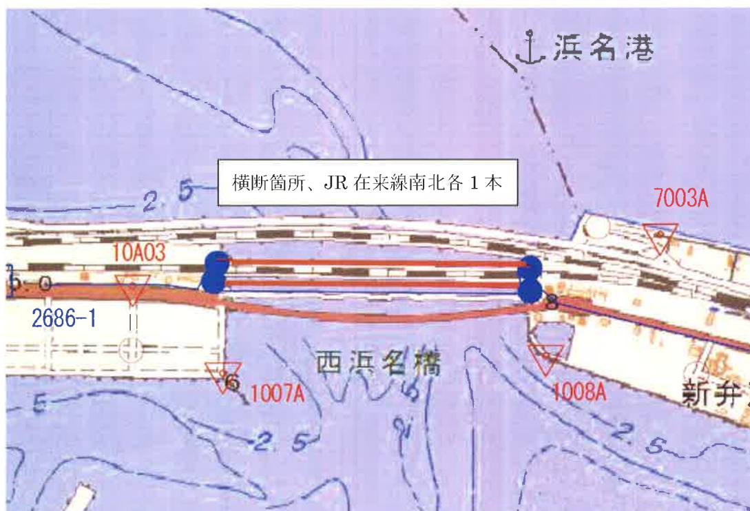
詳細図
