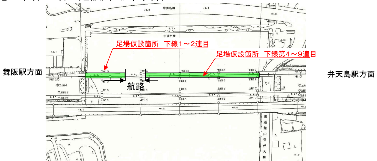
足場平面図
