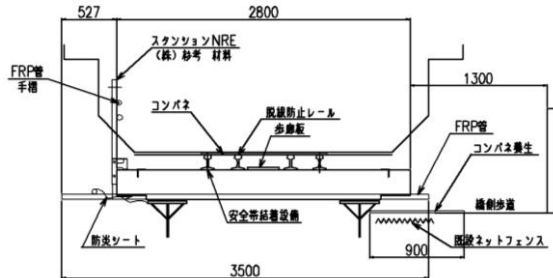
足場断面図
