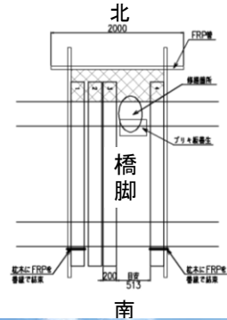
足場平面図
