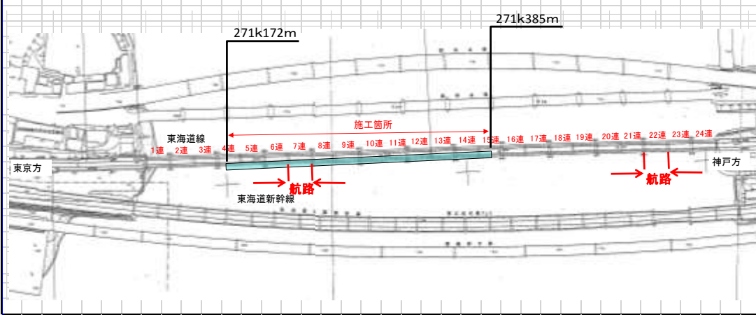
平面図
