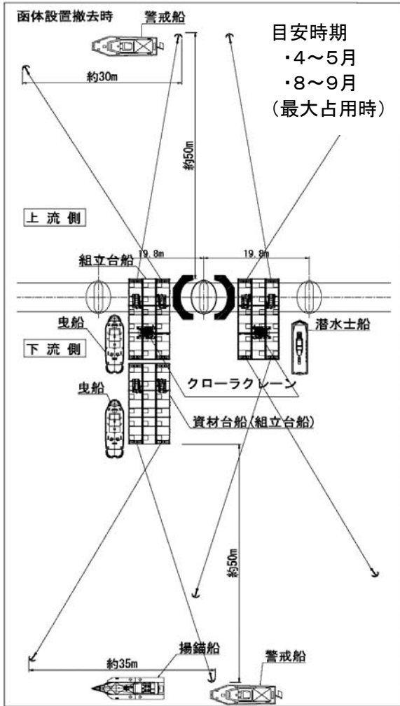
②-1函体設置撤去時イメージ図 目安時期:4~5月・8~9月 (最大占用時)
