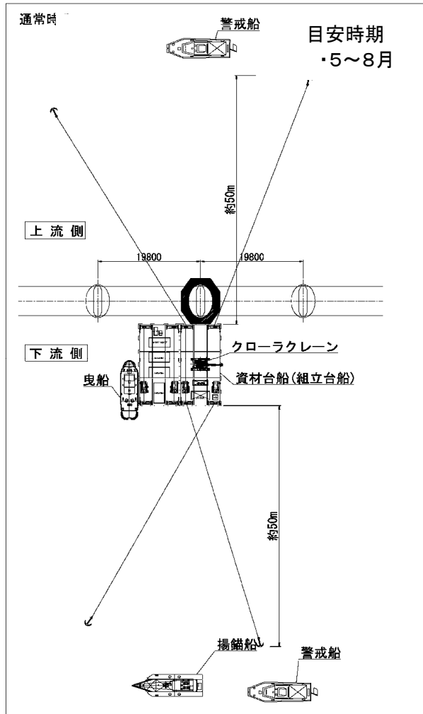
②-2橋脚修繕状況(通常時配置図)
